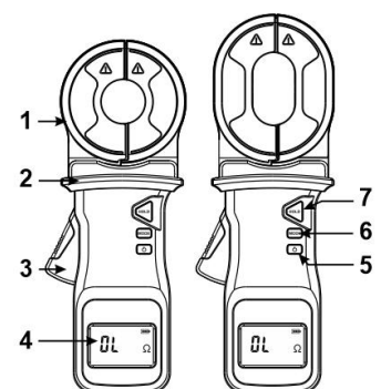
图 1、结构图
